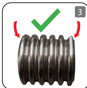
Controleer of de ribbels intact zijn en of er geen vervorming zichtbaar is.
