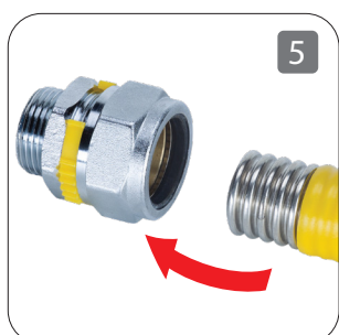
Sluit de slang aan op de fittingen. Belangrijk: zorg dat bij handmatige montage een 'klik' te horen is.
