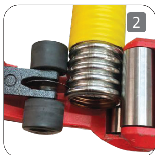
Gebruik indien mogelijk een snijgereedschap met rubberen rolgeleiders en zorg ervoor dat de geleiderollen geen druk uitoefenen op de ribbels van de slang.
