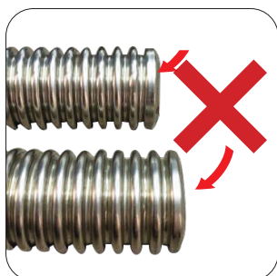
Zorg ervoor dat de ribbels tijdens het snijden niet worden afgeplat of vervormd. Als de ribbelstructuur vervormd is, wordt de correcte werking van de messing ring belemmerd.
