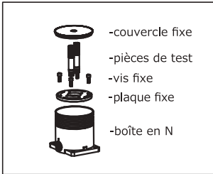
1.VUE ÉCLATÉE BOÎTIER ENCASTRÉ
