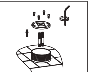
4.Prenez les pièces de rechange, le couvercle, les pièces de test et le gradiomètre.
