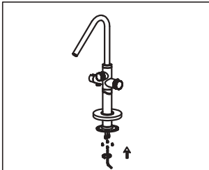
8.Prenez la plaque de fixation et reliez le tuyau à l'aide d'une clé hexagonale H3.
