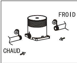
2.Enroulez du ruban téflon autour du raccord, connectez les arrivées d'eau chaude et froide et assurez-vous qu'il n'y ait aucune fuite.
