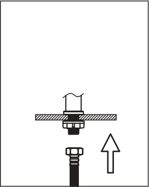
3. Vissez le flexible d’alimentation au robinet.
